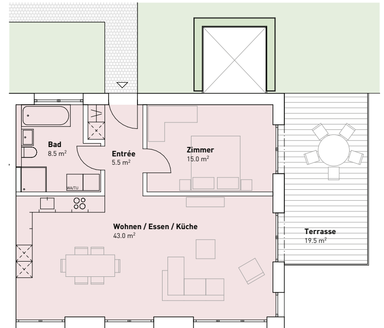
Variante 2.5-Zimmer-Wohnung
